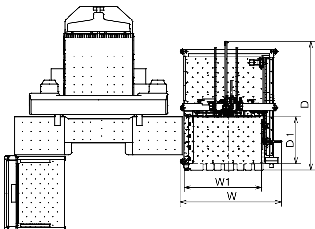
平面寸法図
